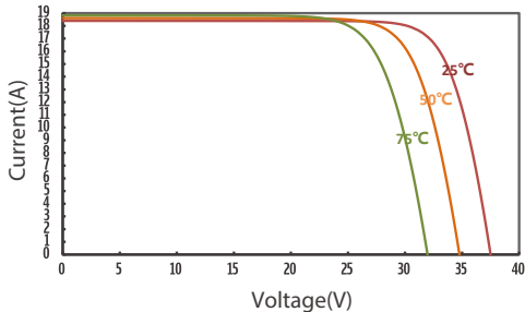
JT550SZk(B) 不同温度下的IV曲线
